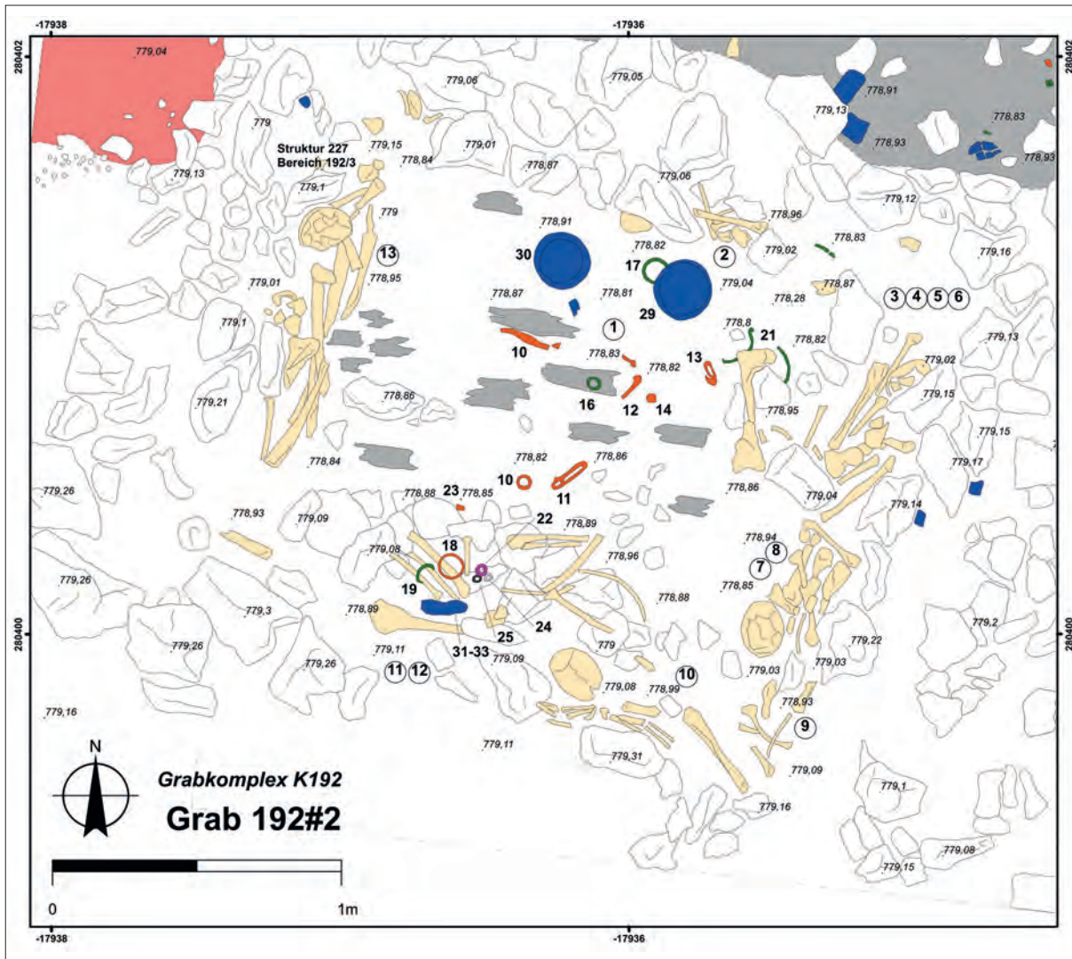
Abb. 7. Hallein, Dürrnberg „Römersteig“, Grab 192#2. Neben den gebündelten und beiseite geräumten skelettierten Menschenresten entlang der Kammerwände könnte der zentrale Freiraum auf die vollständige Entnahme eines Leichnams hinweisen (Dürrnbergforschung KMH).
